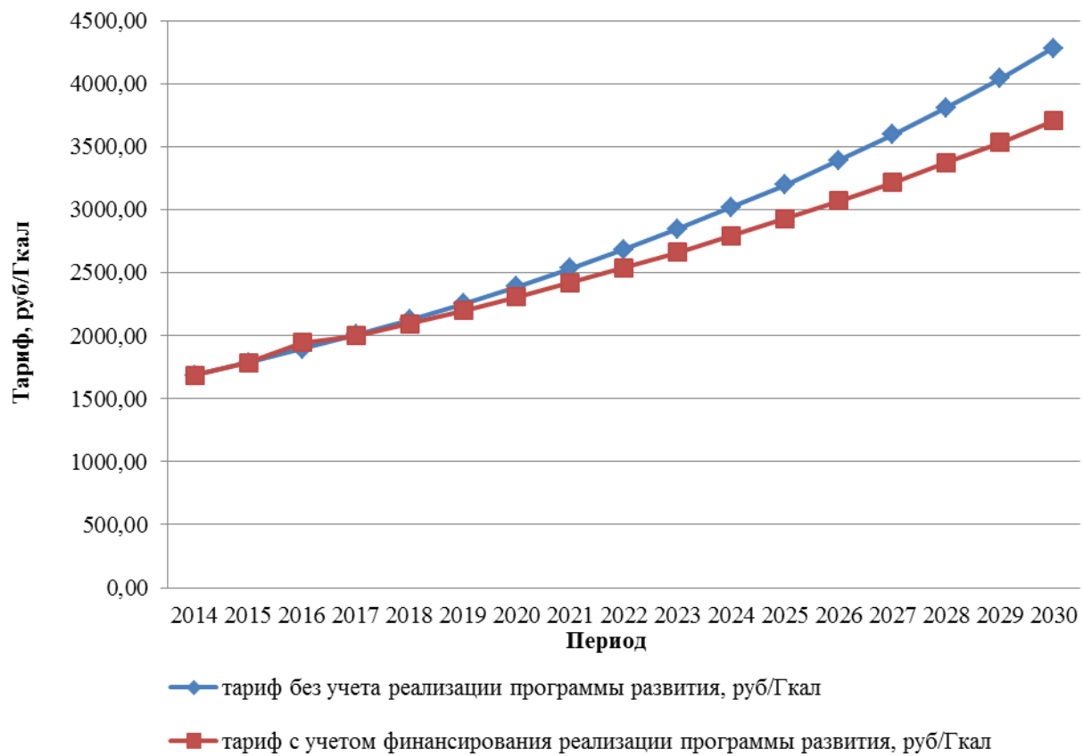
Рисунок 4 – Прогноз величины тарифа по ООО «Ивановское ЖКХ», влияние на величину тарифа реализации мероприятий указанных в программе
